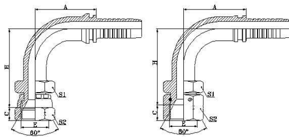
90° 日本公制内螺纹 60° 内锥面 90° JIS METRIC FEMALE 60° CONE SEAT
